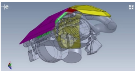
Zaprojektowana obudowa
