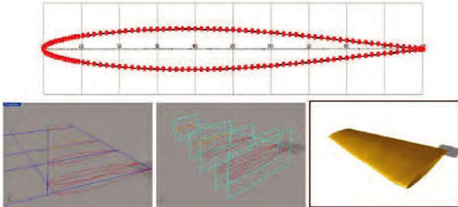
Rys. 15. Etapy rekonstrukcji skrzydła badanego samolotu: profil początkowej części skrzydła NACA64010, poszczególne profile aerodynamiczne na rozpiętości skrzydła oraz krzywe zarysu skrzydła, łączenie poszczególnych profili z krzywymi obrysu skrzydła, gotowy model NURBS skrzydła
