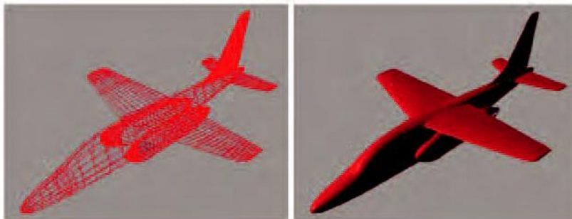
Rys. 16. Zrekonstruowana geometria modelu samolotu do badań flutterowych: siatka głównych krzywych krawędziowych, komputerowy model NURBS
