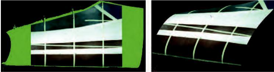
Rys. 4. Kalibracja wielkości chmury punktów (od lewej): pojedyncza chmura punktów wraz z zaznaczonym obszarem do usunięcia (kolor jasnoszary), obrabiona chmura punktów ze skalibrowaną wielkością
